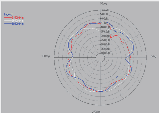
5G (PHI=0)
