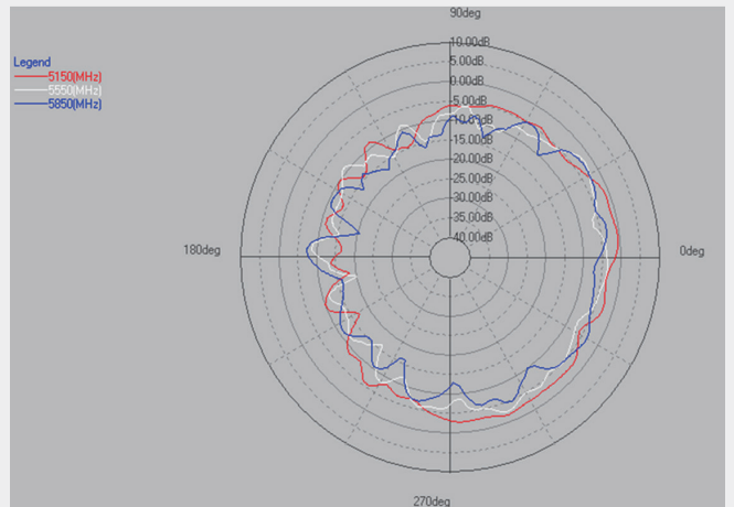
5G (PHI=90)
